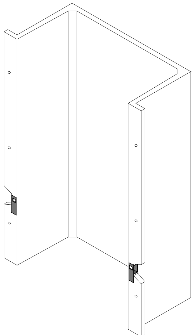
Lichtschacht Optimus 100/50/180 ohne Boden
