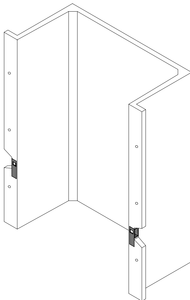
Lichtschacht Optimus 100/50/150 ohne Boden
