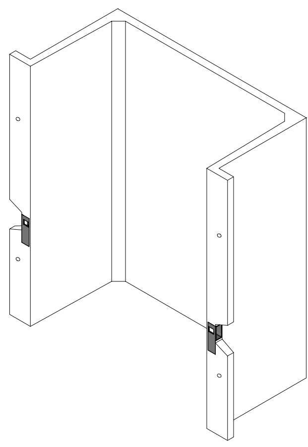
Lichtschaft Optimus 100/50/130 ohne Boden
