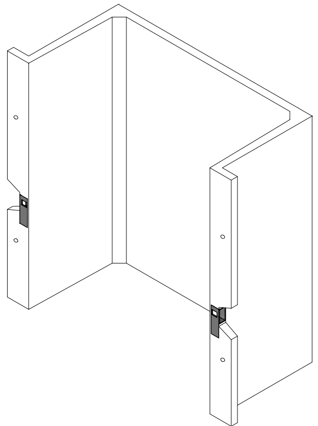
Lichtschacht Optimus 100/50/120 ohne Boden
