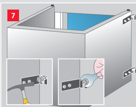
7 Befestigen des Lichtschachts an der Wand mit gleichmäßigen Anpressdruck. Nachklopfen der Dübel und gleichmäßiges Anziehen aller Dübel im Wechsel. Verdichtung des Dichtbandes auf 20% (ca. 5-6 mm)
